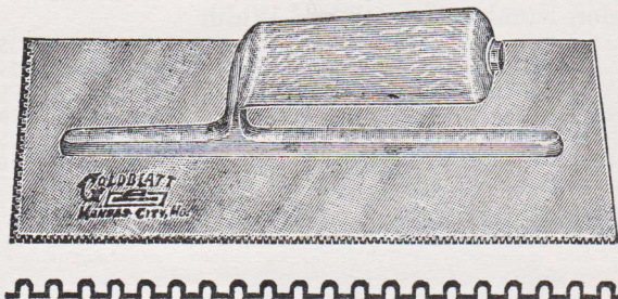
Actual Size of Notches in Trowel No. 55-S
